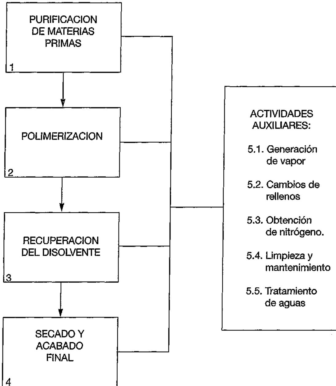
FIGURA 1: DIAGRAMA GENERAL DEL PROCESO
