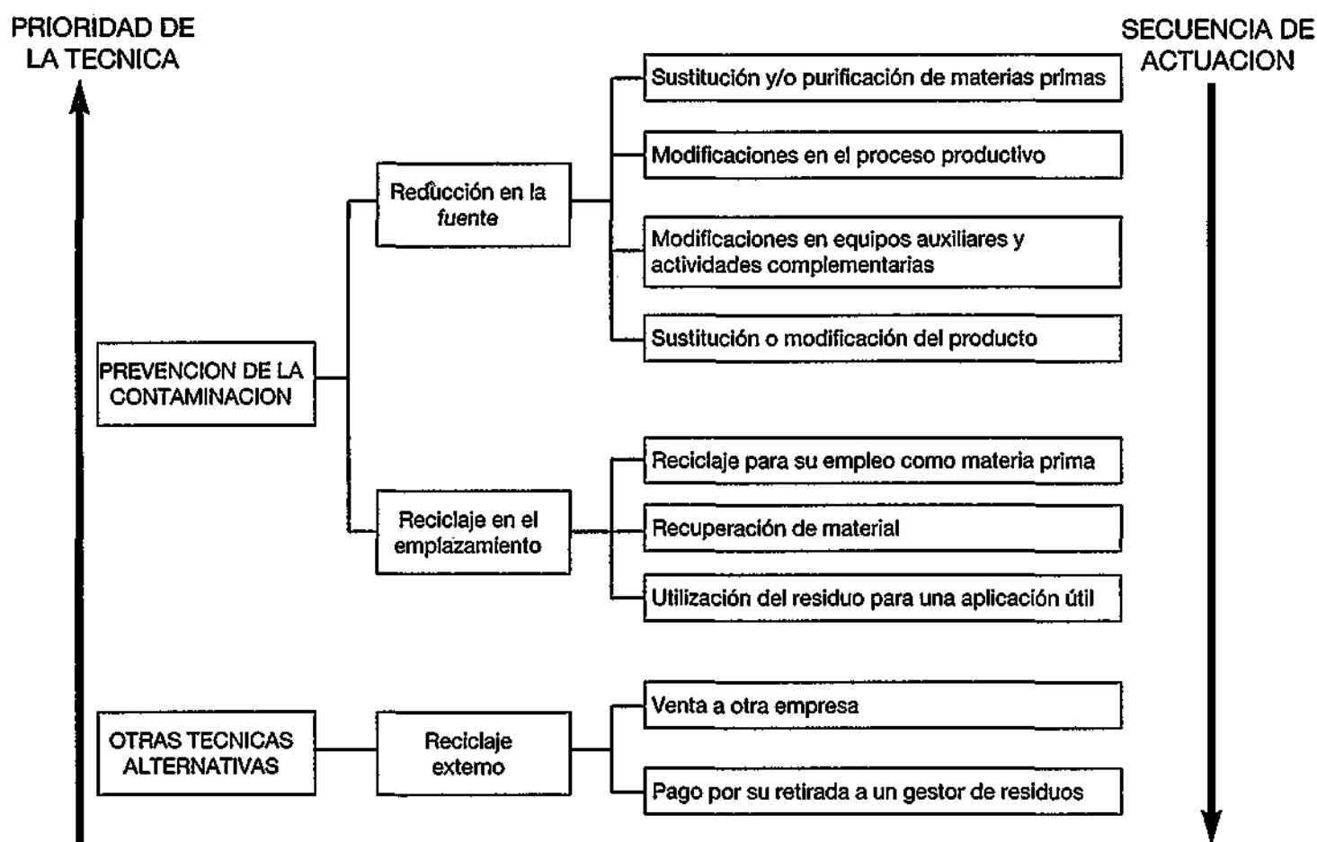
FIG. 1: TECNICAS DE MINIMIZACION DE LA CONTAMINACION
