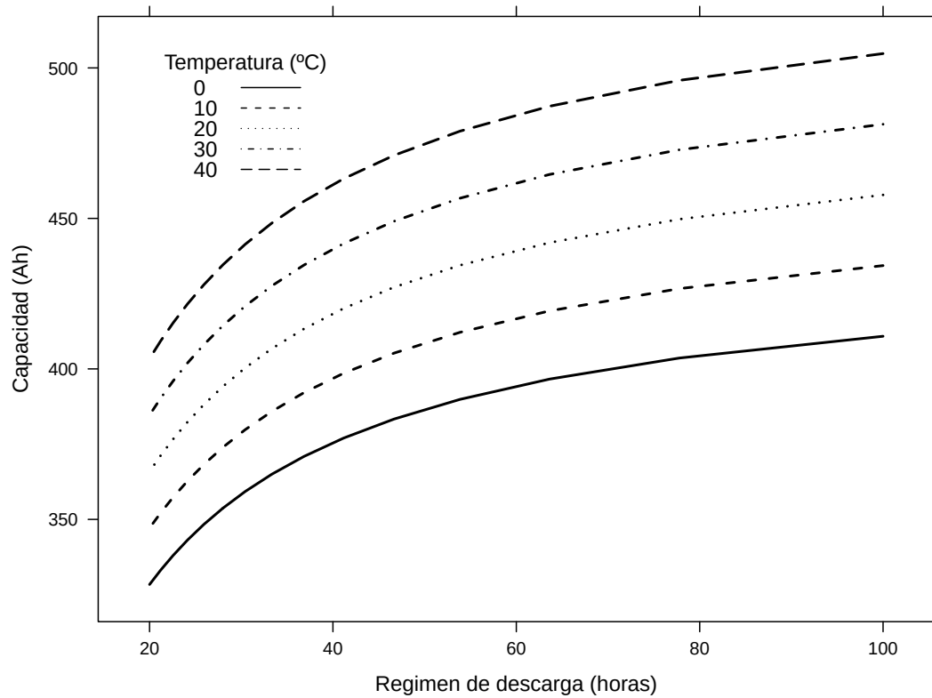
FIGURA 7.5: Relación entre el régimen de descarga y la capacidad de la batería.
