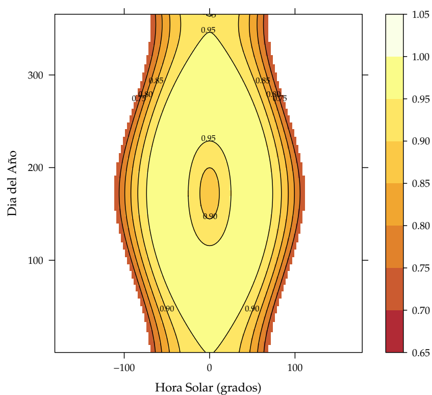
FIGURA 2.18: Coseno del ángulo de incidencia de un seguidor acimutal a lo largo del día y año para un sitio con latitud 40°N.
