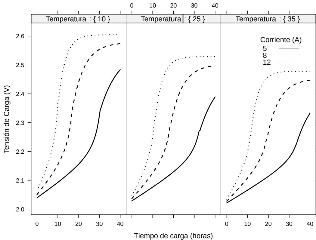
FIGURA 7.3: Curvas de evolución de la tensión en bornes de una batería durante un proceso de carga a corriente constante, para diferentes valores de corriente de carga y temperatura ambiente. Las curvas están particularizadas para una batería con una capacidad C_{10} = 300 Ah. Se ha utilizado el modelo de comportamiento propuesto en la referencia [31].
