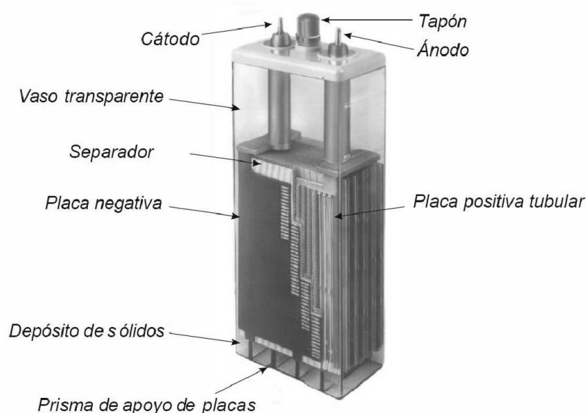
FIGURA 7.6: Batería estacionaria con desglose de elementos.
