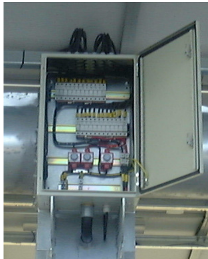
FIGURA 9.12: Caja de protección DC. Incluye dos fusibles por rama y varistores entre polos y tierra.
