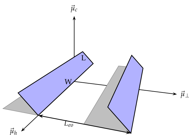
FIGURA 6.16: Dimensiones básicas en sistemas con seguidores de eje horizontal.
