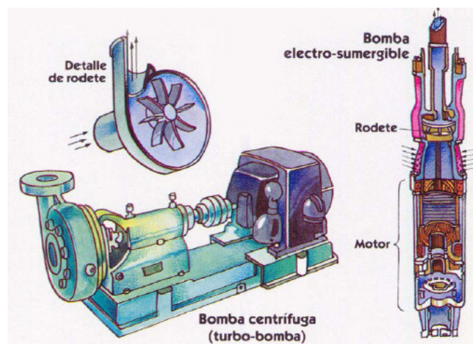
FIGURA 8.4: Bomba centrífuga de superficie y sumergible.
