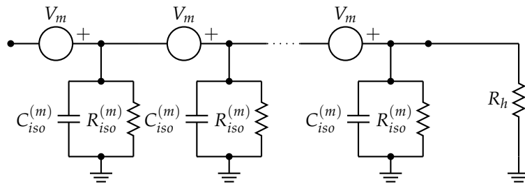
FIGURA 9.4: Capacidad distribuida en un generador fotovoltaico con esquema de conexión a tierra IT.
