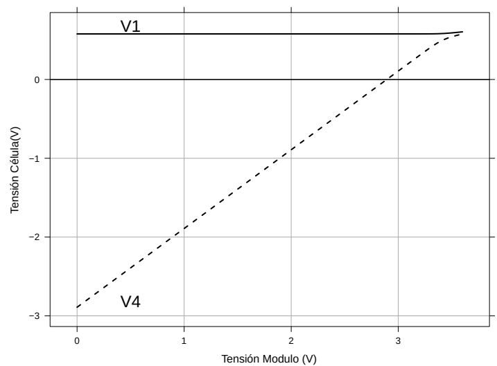
FIGURA 5.2: Tensión de las células 1 y 4 para diferentes tensiones del módulo definido por la agrupación serie de la figura 5.1.
