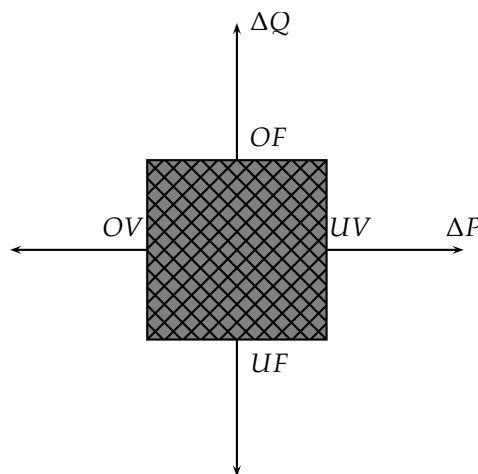
FIGURA 6.6: Zona de no detección en modo isla. Cualquier combinación de potencia activa y reactiva de red antes de la desconexión que se encuentre dentro de esa región implica que el inversor continuaría funcionando en modo isla durante un tiempo.
