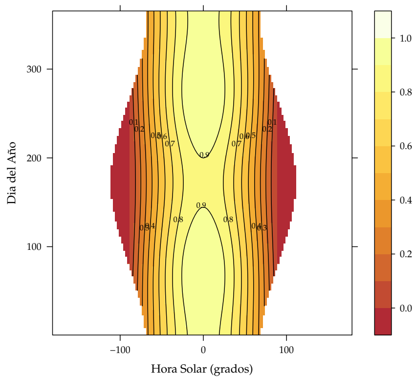
FIGURA 2.13: Coseno del ángulo de incidencia en un sistema estático a lo largo del día y año para un sitio con latitud 40^\circ\text{N} .
