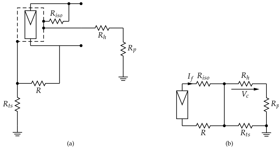
FIGURA 9.6: Esquema eléctrico de contacto indirecto en un sistema fotovoltaico con esquema de conexión a tierra TN.
