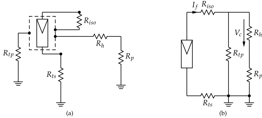
FIGURA 9.5: Esquema eléctrico de contacto indirecto en un sistema fotovoltaico con esquema de conexión a tierra TT.
