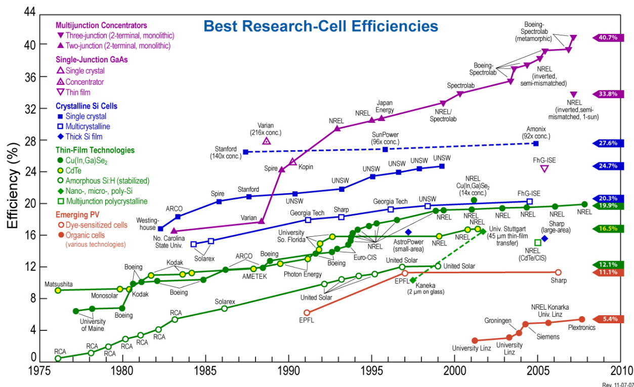
FIGURA 4.7: Evolución de la eficiencia de células según la tecnología (según el National Renewable Energy Laboratory (EEUU)).
