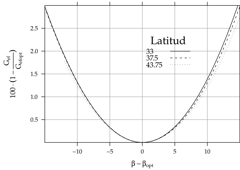
FIGURA 3.9: Pérdidas de irradiación global anual al elegir un ángulo de inclinación diferente del óptimo para tres latitudes diferentes en el hemisferio Norte.
