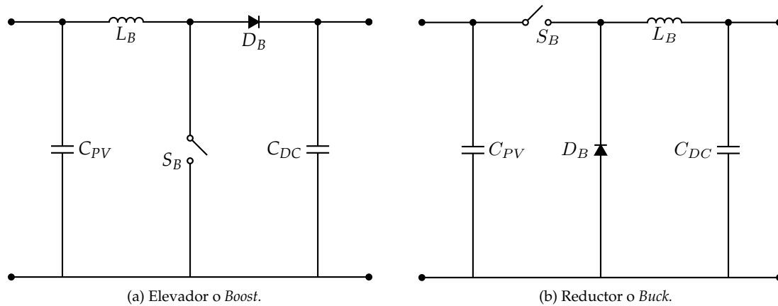
FIGURA 8.5: Convertidores DC-DC.
