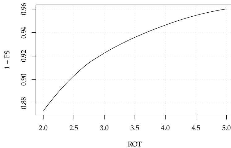
FIGURA 6.17: Separación entre seguidores de eje horizontal.
