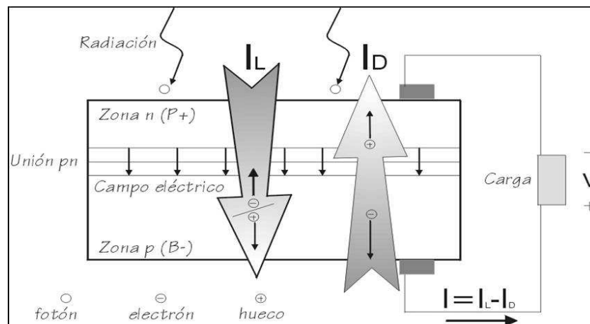
FIGURA 4.4: Corriente de iluminación y corriente de diodo en una célula solar que alimenta a una carga.
