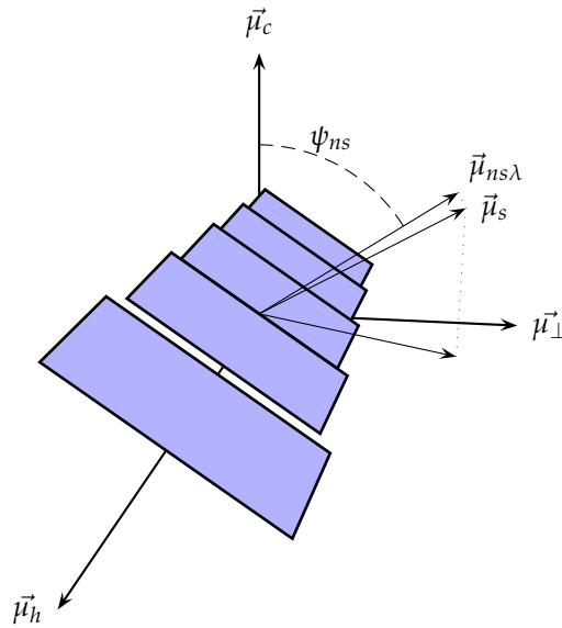
FIGURA 2.16: Lamas inclinadas en seguidor de eje horizontal Norte-Sur.
