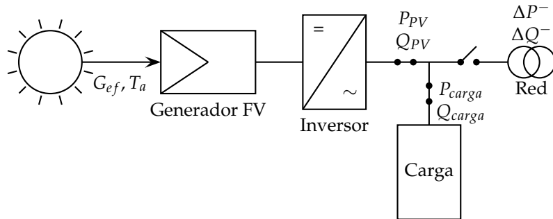
FIGURA 6.5: Sistemas fotovoltaicos conectados a barra de distribución.
