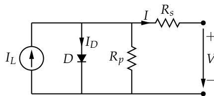
FIGURA 4.10: Modelo eléctrico de una célula solar.
