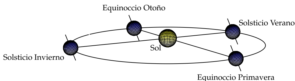
FIGURA 2.1: Trayectoria Sol-Tierra. Los nombres de los solsticios y equinoccios están particularizados para el hemisferio Norte.
