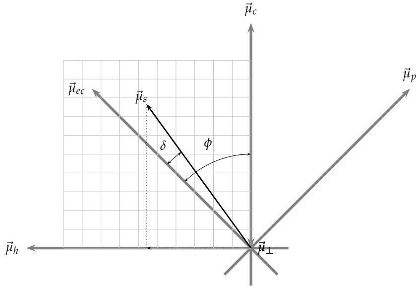
FIGURA 2.7: Relación entre los sistemas de coordenadas terrestre y local (particularizado para el hemisferio Norte).
