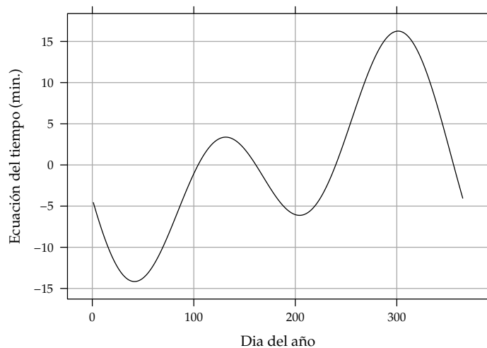
FIGURA 2.11: Ecuación del tiempo (minutos)
