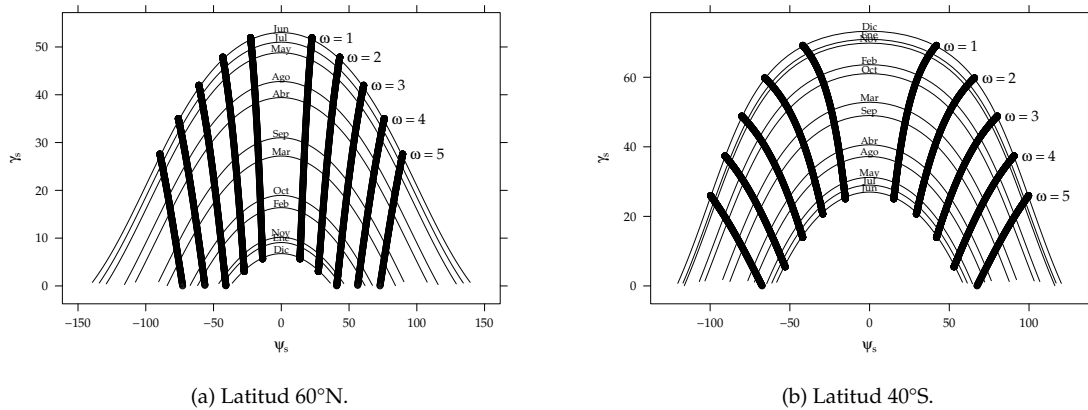
FIGURA 2.9: Diagrama de trayectoria solar según los ángulos de elevación y acimut en dos localidades terrestres.
