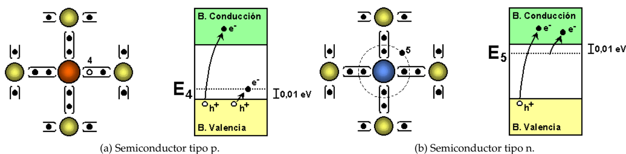
FIGURA 4.1: Semiconductores dopados.
