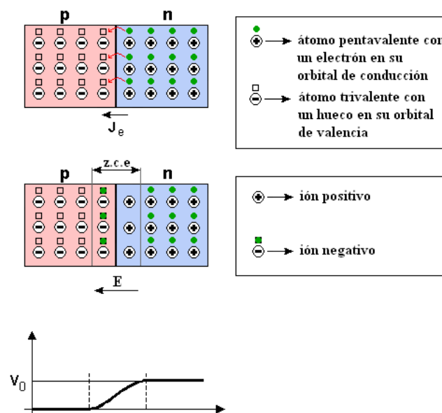
FIGURA 4.2: Unión p-n..
