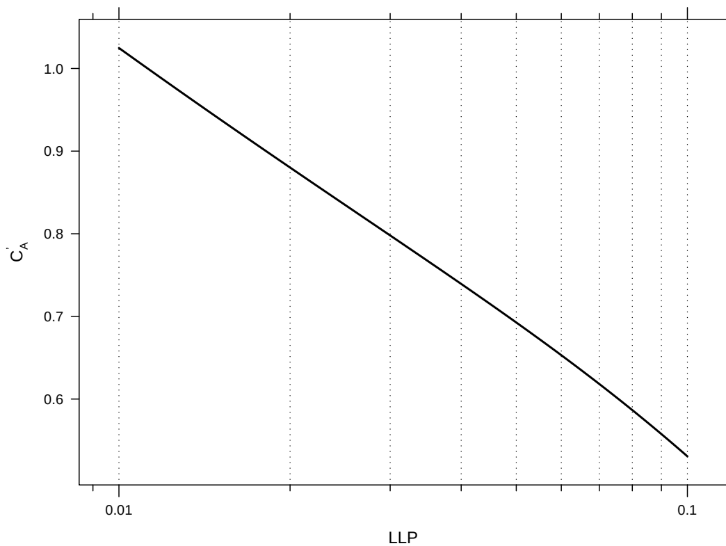
FIGURA 7.10: Relación entre C'_A y LLP para C_S = 3 (escala logarítmica en LLP).
