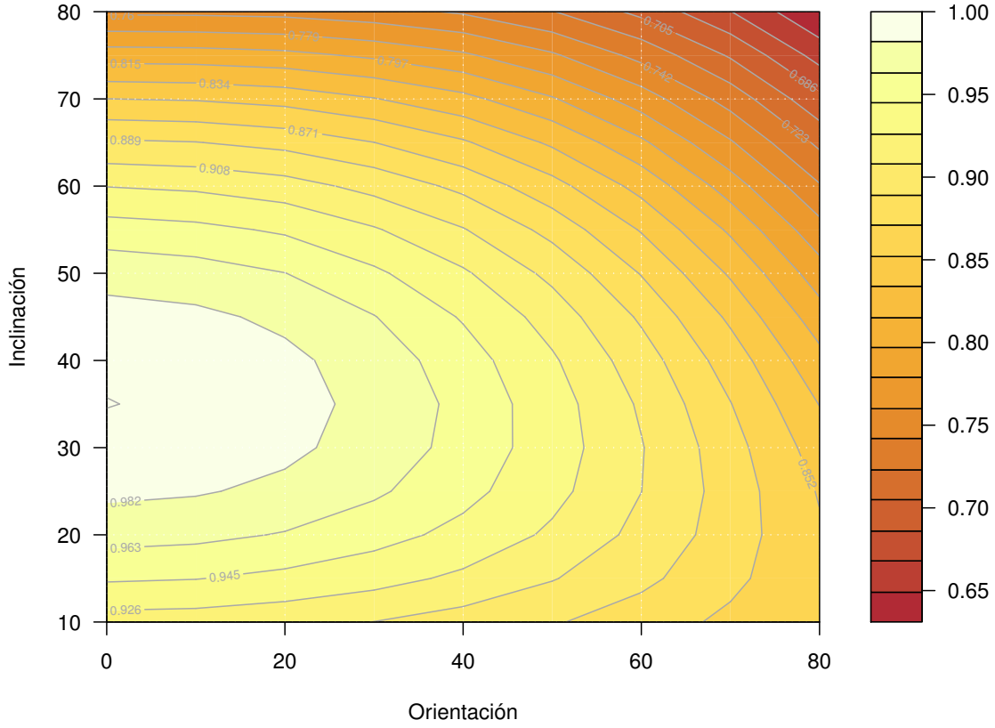
FIGURA 6.7: Energía producida por un SFCR con una orientación e inclinación determinada respecto a la energía producida por el mismo SFCR con la orientación e inclinación óptimas.
