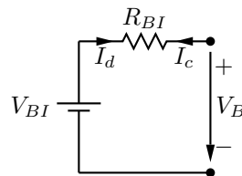
FIGURA 7.2: Modelo eléctrico de batería.
