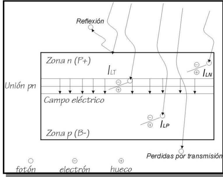
FIGURA 4.5: Pérdidas de transmisión, reflexión y recombinación en una célula solar.
