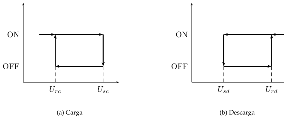
FIGURA 7.8: Histéresis de protección frente a sobrecarga y sobredescarga en un regulador.
