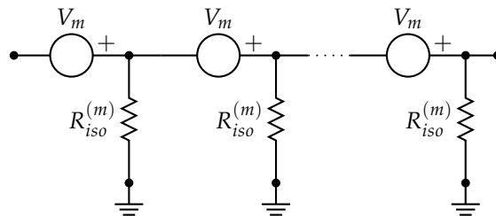
FIGURA 9.3: Resistencia de aislamiento distribuida en un generador fotovoltaico con esquema de conexión a tierra IT.
