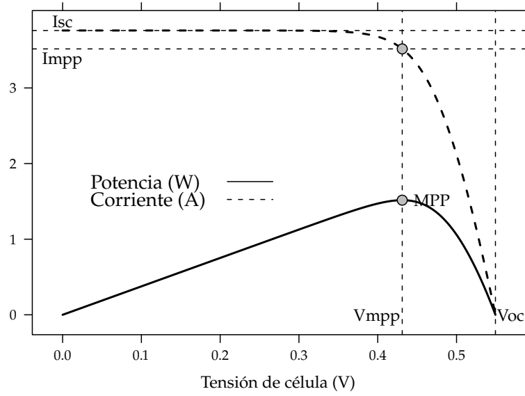
FIGURA 4.6: Curvas corriente-tensión (línea discontinua) y potencia-tensión (línea continua) de una célula solar ( T_a = 20^\circ\text{C} y G = 800\text{ W/m}^2 ).
