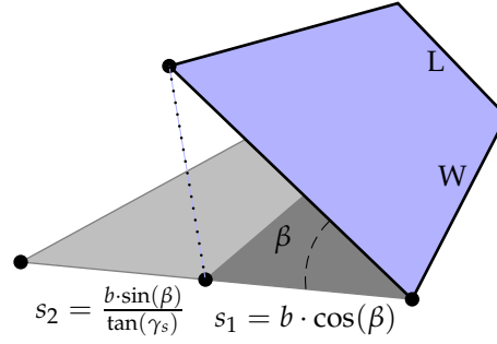
FIGURA 6.12: Dimensiones de un seguidor a doble eje y longitud de su sombra arrojada.
