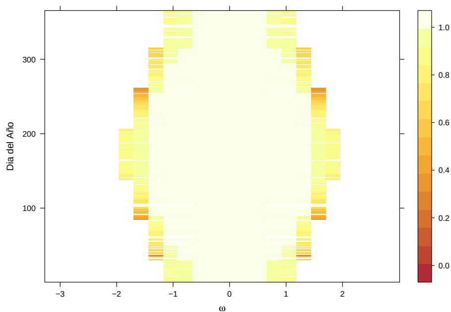
FIGURA 6.15: Evolución del sombreado en un seguidor promedio situado en una cuadrícula. En la gráfica, el valor 0 indica sombra total y el valor 1 ausencia de sombra.
