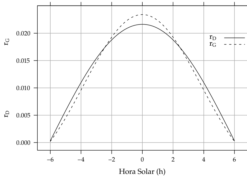
FIGURA 3.4: Perfil de irradiancia difusa y global obtenido a partir del generador empírico de [29] para valores de irradiancia tomadas cada 10 minutos.
