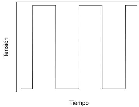
FIGURA 6.3: Evolución temporal de una onda cuadrada de tensión empleada para controlar conmutación de un inversor.
