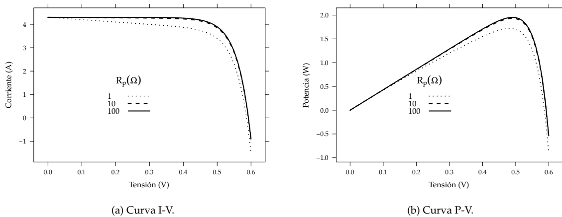
FIGURA 4.9: Efecto de la resistencia paralelo en las curvas I-V y P-V.
