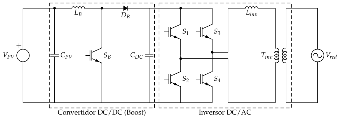
FIGURA 6.2: Esquema de un inversor monofásico con topología VSI. La figura incluye un convertidor DC/DC tipo Boost (elevador) junto con el puente inversor, ambos utilizando dispositivos IGBTs. Este equipo incluye un transformador de baja frecuencia a la salida.
