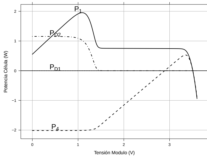
FIGURA 5.7: Potencias de los elementos de la figura 5.4 para diferentes tensiones de la agrupación serie.
