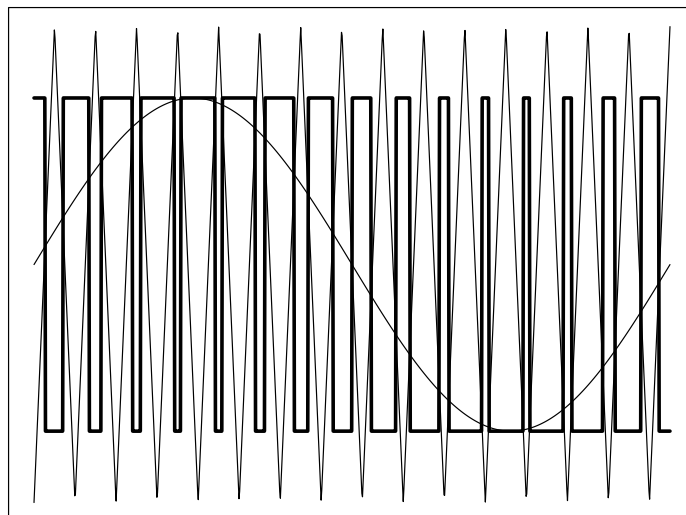
FIGURA 6.4: Onda SPWM monofásica bipolar.
