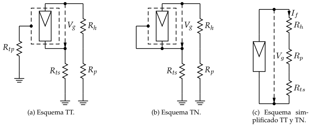
FIGURA 9.2: Esquema eléctrico de un contacto directo en un sistema fotovoltaico con esquema de puesta a tierra TT o TN.
