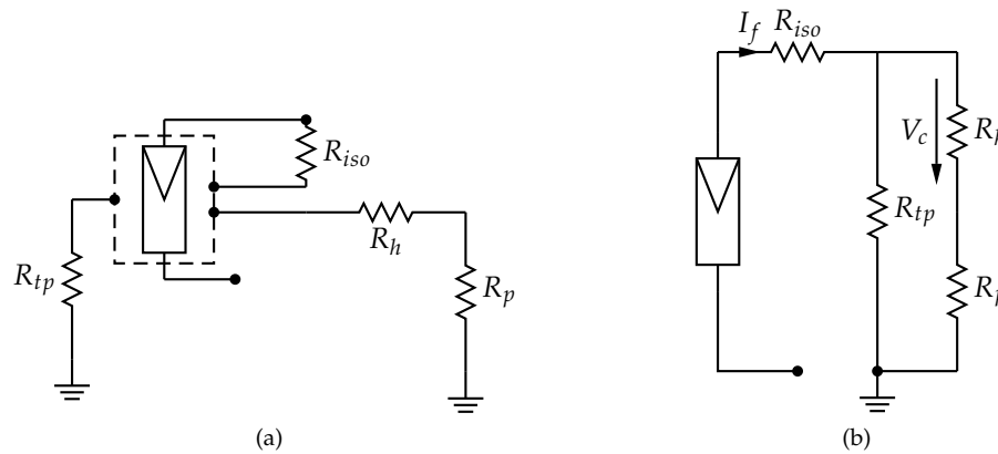
FIGURA 9.7: Esquema eléctrico de contacto indirecto en un sistema fotovoltaico con esquema de conexión a tierra IT.
