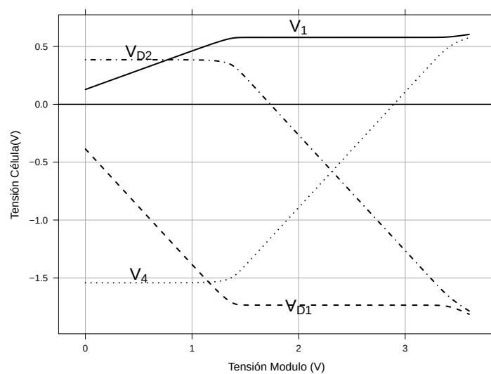
FIGURA 5.6: Tensiones en los elementos de la figura 5.4 para diferentes tensiones de la agrupación serie.
