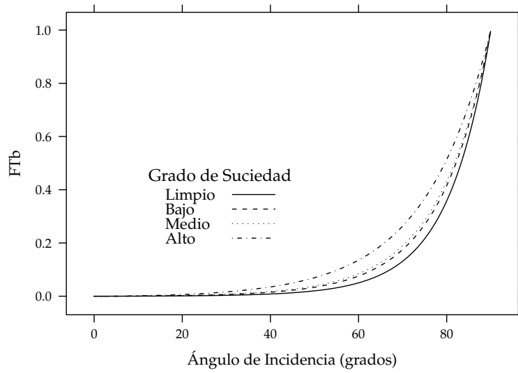
FIGURA 3.7: Pérdidas angulares de un módulo fotovoltaico para diferentes grados de suciedad en función del ángulo de incidencia.
