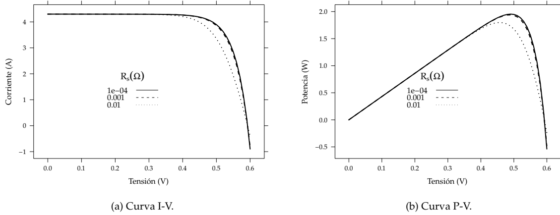
FIGURA 4.8: Efecto de la resistencia serie en las curvas I-V y P-V.
