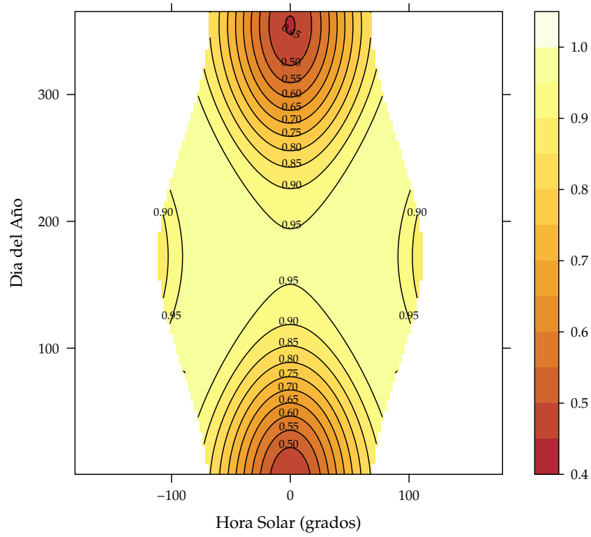
FIGURA 2.15: Coseno del ángulo de incidencia en un sistema de eje horizontal Norte-Sur a lo largo del día y año para un sitio con latitud 40°N.
