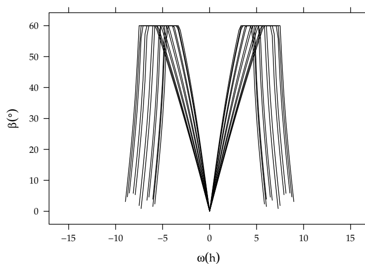
FIGURA 6.18: Retroseguimiento y limitación del ángulo de inclinación en seguidores de eje horizontal.
