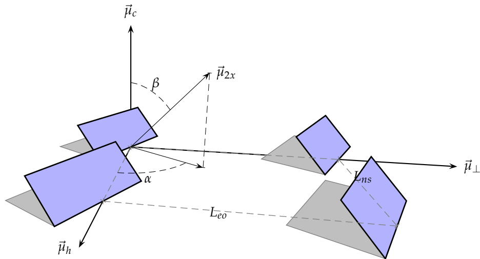
FIGURA 6.11: Sombras mutuas en un conjunto de cuatro seguidores.
