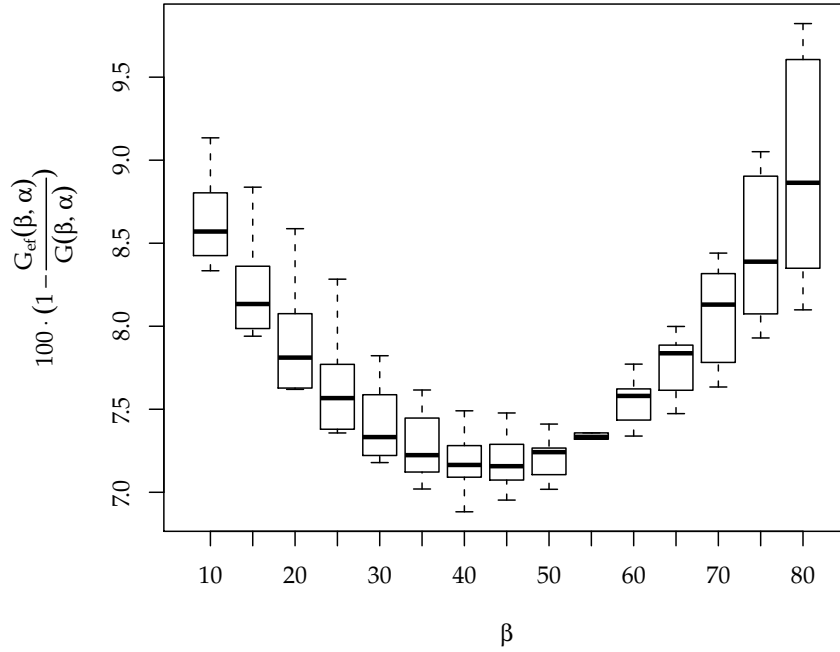
FIGURA 3.8: Pérdidas por suciedad e incidencia no perpendicular integradas a lo largo de un año en Madrid, para un grado de suciedad medio, y para diferentes ángulos de inclinación y orientación.
