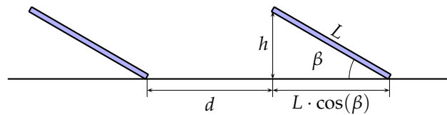
FIGURA 6.10: Dimensiones y distancias entre filas de un sistema estático.
