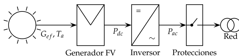
FIGURA 6.1: Esquema de un SFCR.
