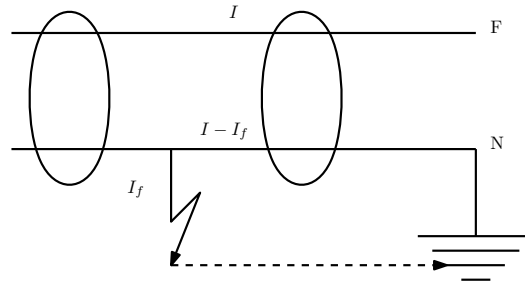
FIGURA 9.13: Funcionamiento de un interruptor diferencial.
