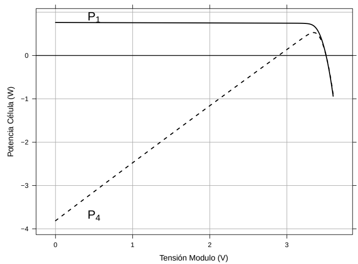
FIGURA 5.3: Potencia de las células 1 y 4 para diferentes tensiones del módulo definido por la agrupación serie de la figura 5.1.
