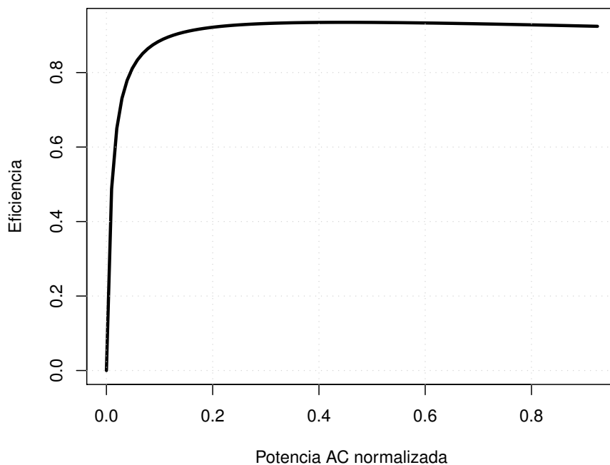
FIGURA 6.8: Curva de eficiencia de un inversor calculada con tres coeficientes genéricos ( k_0^o = 0,01 , k_1^o = 0,025 , k_2^o = 0,05 ).
