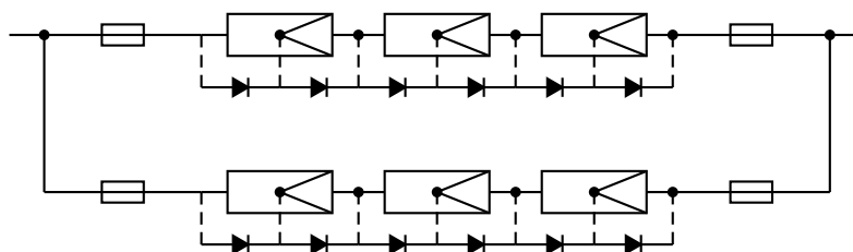
FIGURA 5.10: Esquema de un generador fotovoltaico compuesto por 2 ramas de 3 módulos en serie. El esquema incluye la protección con fusibles y por rama y los diodos de paso incluidos en cada módulo.
