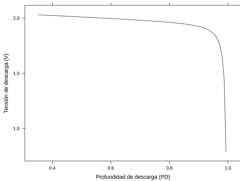
FIGURA 7.4: Relación entre la tensión y la profundidad de descarga de una batería para un proceso de descarga a corriente constante. Esta curva está particularizada para un régimen de descarga de 100 h y temperatura ambiente de 25 °C, para una batería con capacidad C_{10} = 300 Ah.
