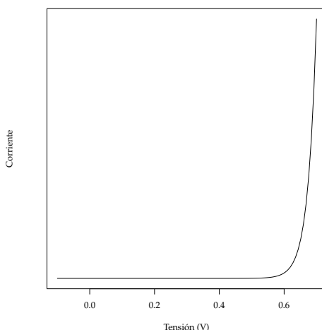
(a) Característica corriente-tensión de un diodo según la ecuación 4.1.
