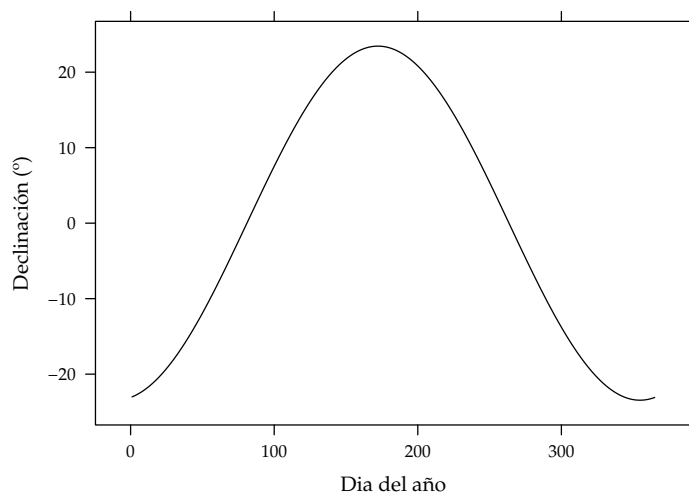
FIGURA 2.2: Declinación.
