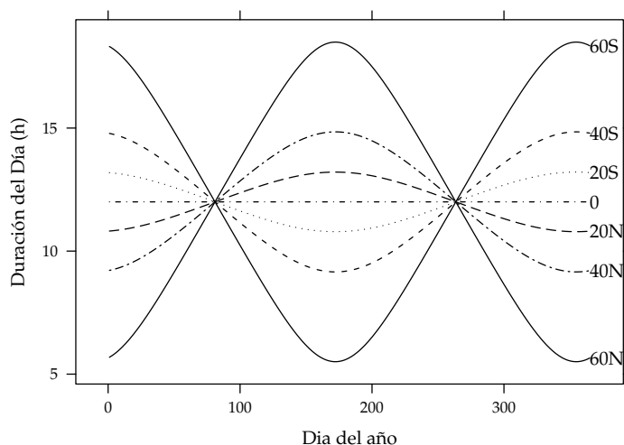
FIGURA 2.10: Duración del día en diferentes latitudes.
