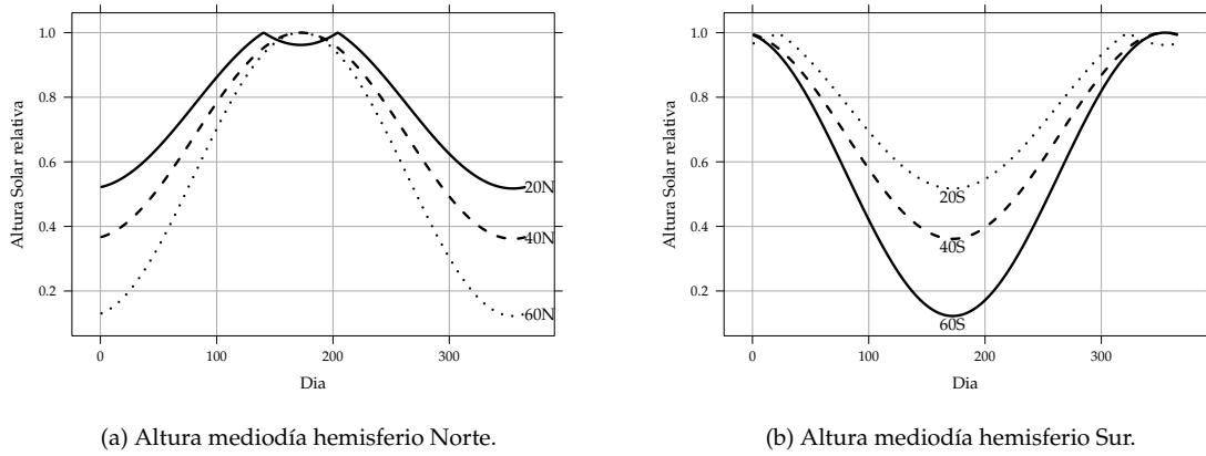
FIGURA 2.8: Altura relativa al mediodía a lo largo del año.
