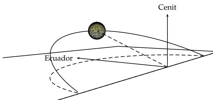
FIGURA 2.5: Movimiento aparente del Sol desde un lugar de la Tierra.
