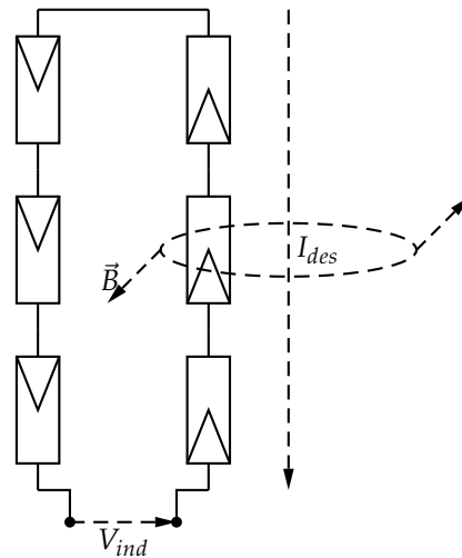
FIGURA 9.9: Inducción sobre un generador.
