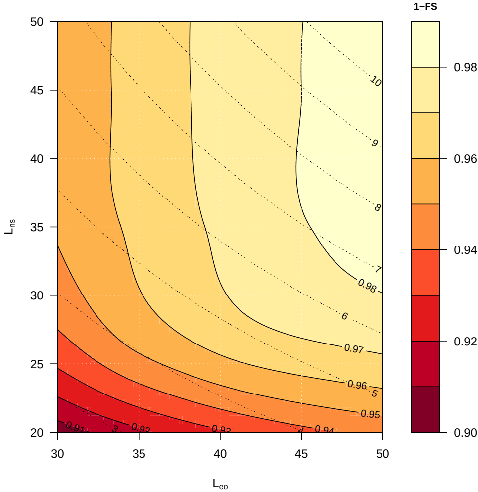
FIGURA 6.14: Ábaco para planta de seguimiento a doble eje. Recoge el ratio entre la energía anual producida por un seguidor afectado por sombras mutuas ( E_{acS} ) y la producida por un seguidor sin sombreado ( E_{ac0} ). Las curvas de color negro representan la fracción de energía no afectada por sombras. Las curvas de puntos representan el valor del ROT.
