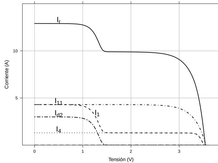
FIGURA 5.5: Curva corriente-tensión de la agrupación serie de la figura 5.4. La corriente I_{11} representa la corriente que circularía por la célula C_1 si la célula C_4 no presentase problemas.
