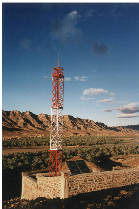
FIGURA 1.3: Sistema fotovoltaico autónomo alimentando un radioenlace.
