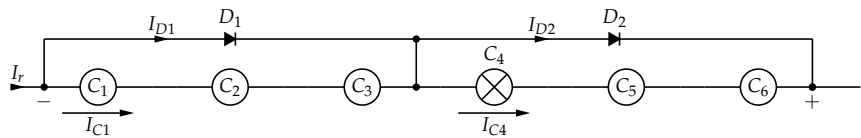
FIGURA 5.4: Colocación de diodo de paso para evitar el fenómeno de punto caliente.
