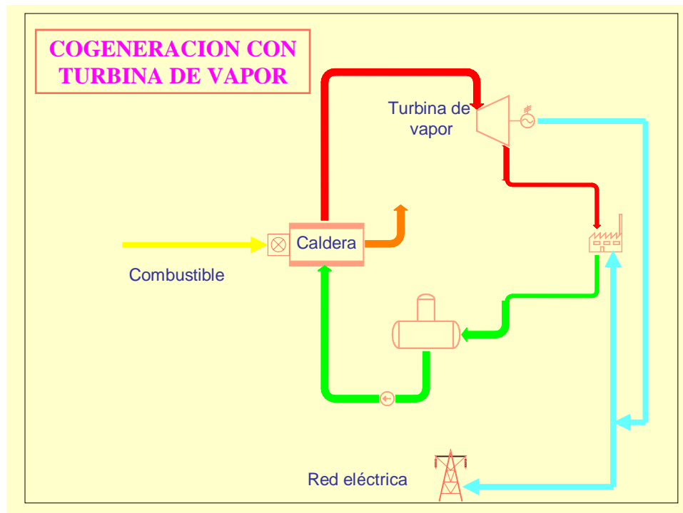
FIG. I.7. PLANTA DE COGENERACIÓN CON TURBINA DE VAPOR
