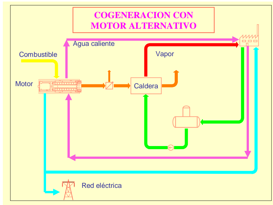
FIG. I.3. PLANTA DE COGENERACIÓN CON MOTOR ALTERNATIVO
