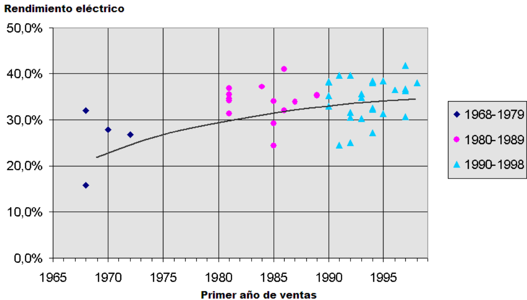
FIG VIII.1. EVOLUCIÓN HISTÓRICA DEL RENDIMIENTO MEDIO DE LAS TURBINAS DE GAS.
