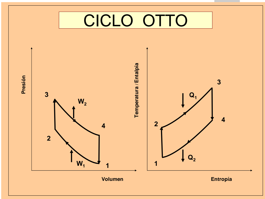
FIG. III.3. CICLO OTTO. DIAGRAMAS P-V Y T-S
