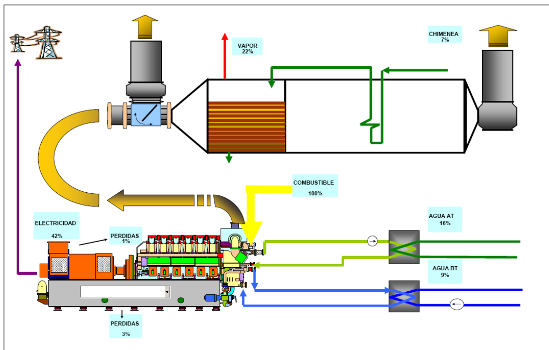
FIG . III.3. BALANCE DE ENERGÍA EN UNA INSTALACIÓN DE MOTOR DE GAS CON CALDERA DE RECUPERACIÓN
