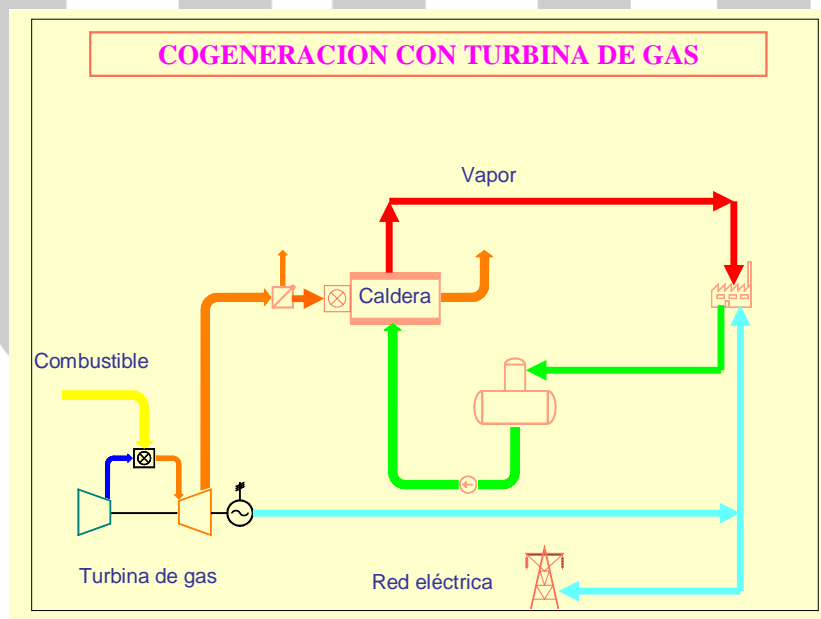
FIG. I.5. PLANTA DE COGENERACIÓN CON TURBINA DE GAS
