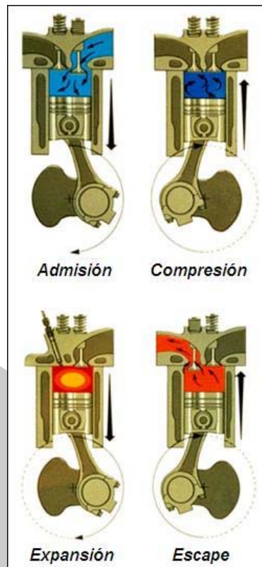
FIG III.2. FASES EN UN MOTOR ALTERNATIVO DE CUATRO TIEMPOS
