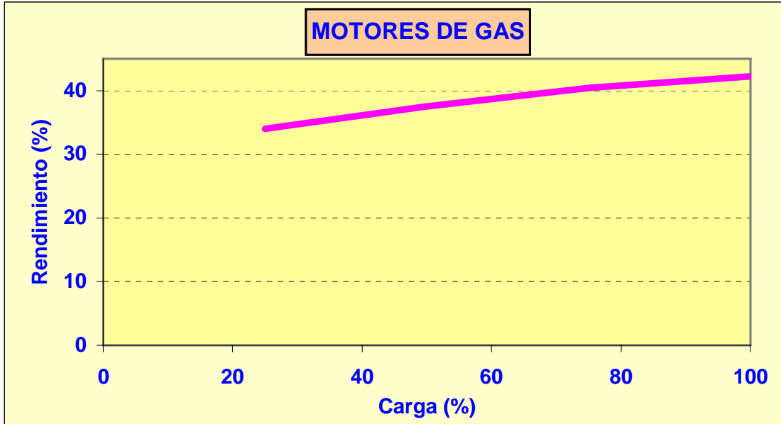
FIG VII.4. VARIACIÓN DEL RENDIMIENTO DE UN MOTOR DE GAS CON LA CARGA
