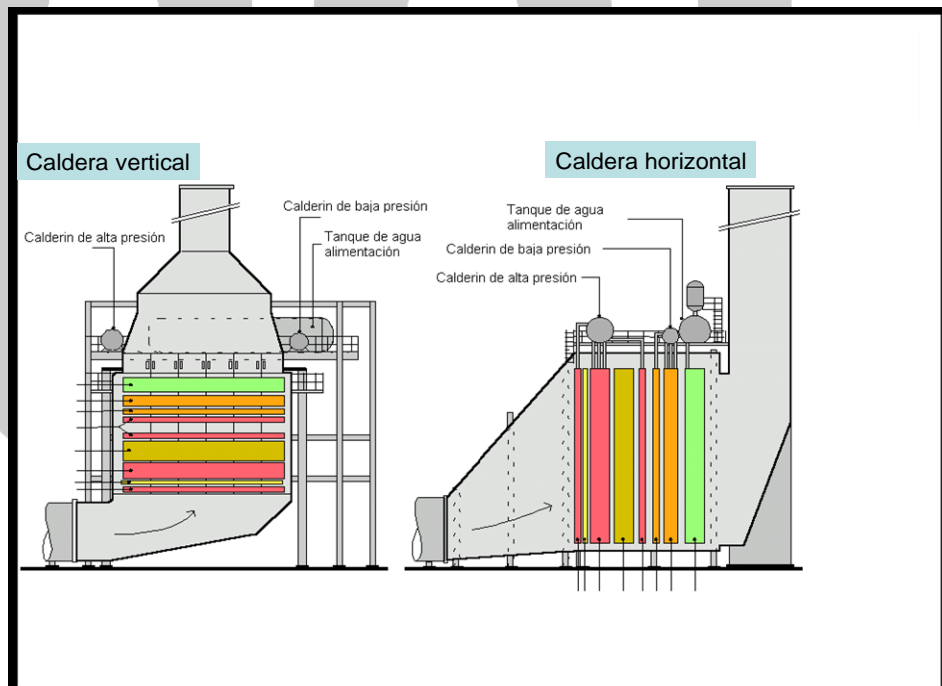
FIG IV.1. DISPOSICIONES DE CALDERAS ACUOTUBULARES
