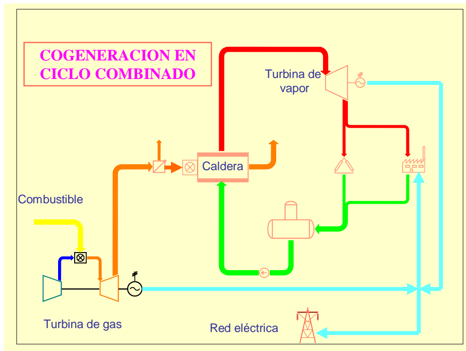
FIG. I.8. PLANTA DE COGENERACIÓN EN CICLO COMBINADO CON TURBINA DE GAS
