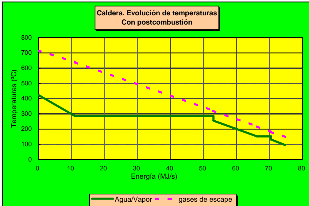
FIG VIII.5. EVOLUCIÓN DE TEMPERATURAS DE AGUA-VAPOR Y GASES DE ESCAPE, EN UNA CALDERA DE RECUPERACIÓN DE CALOR CON DOS NIVELES DE PRESIÓN, CUANDO SE TRABAJA CON POSTCOMBUSTIÓN.
