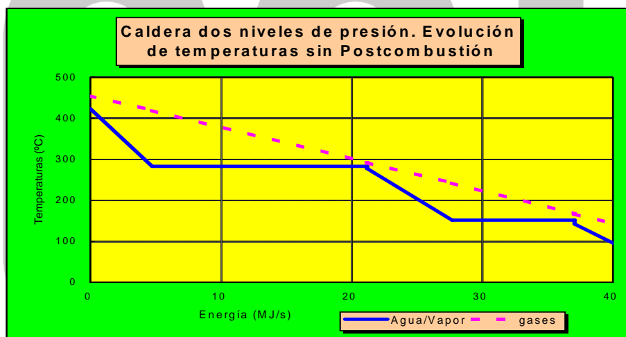
FIG. VIII.4. EVOLUCIÓN DE TEMPERATURAS DE AGUA-VAPOR Y GASES DE ESCAPE, EN UNA CALDERA DE RECUPERACIÓN DE CALOR CON DOS NIVELES DE PRESIÓN
