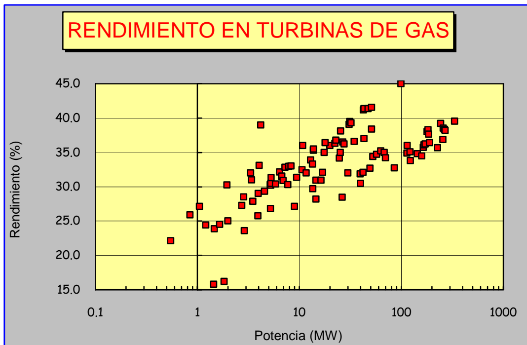
FIG VIII.2. VARIACIÓN DEL RENDIMIENTO CON EL TAMAÑO DE LAS TURBINAS DE GAS
