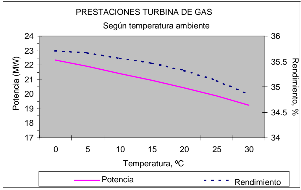
FIG VIII.6. VARIACIÓN DE LAS PRESTACIONES DE UNA TURBINA DE GAS DE 22 MW CON LA TEMPERATURA AMBIENTE.
