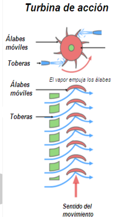
FIG II.1 FUNCIONAMIENTO ESQUEMÁTICO DE UNA TURBINA DE ACCIÓN
