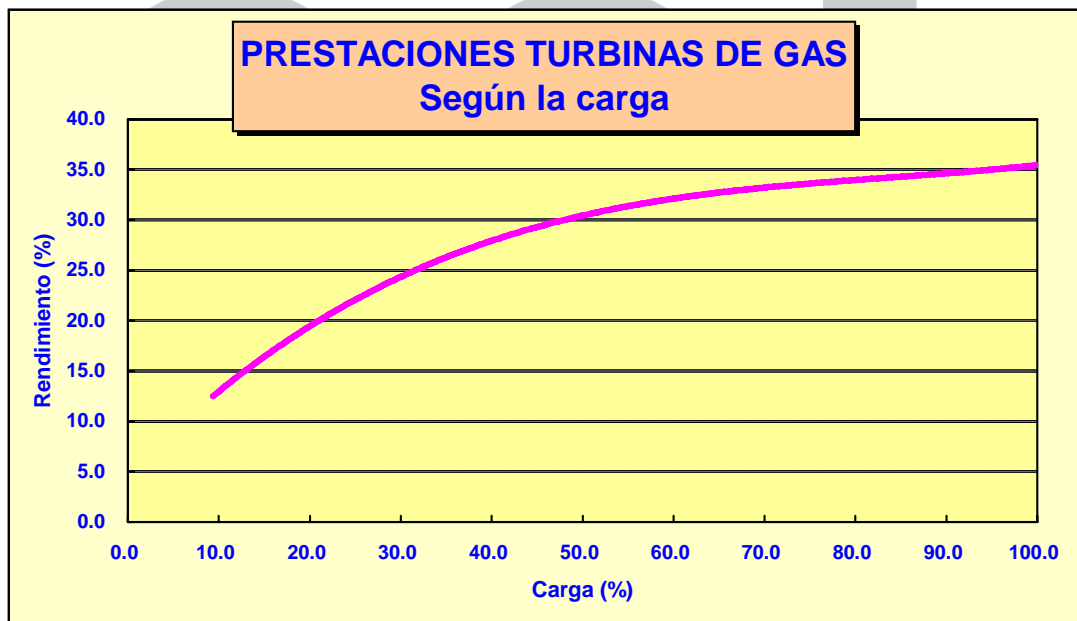
FIG VII.5. VARIACIÓN DEL RENDIMIENTO DE UNA TURBINA DE GAS CON LA CARGA
