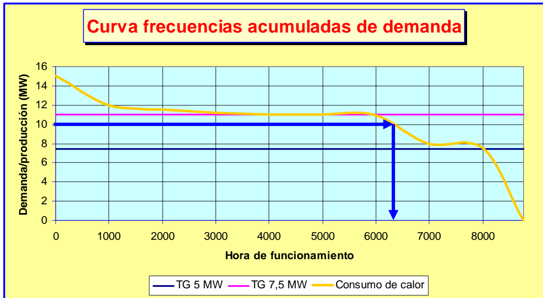
FIG VII.10 COMPARACIÓN CAPACIDAD DE PLANTA CON DEMANDA DE CALOR
