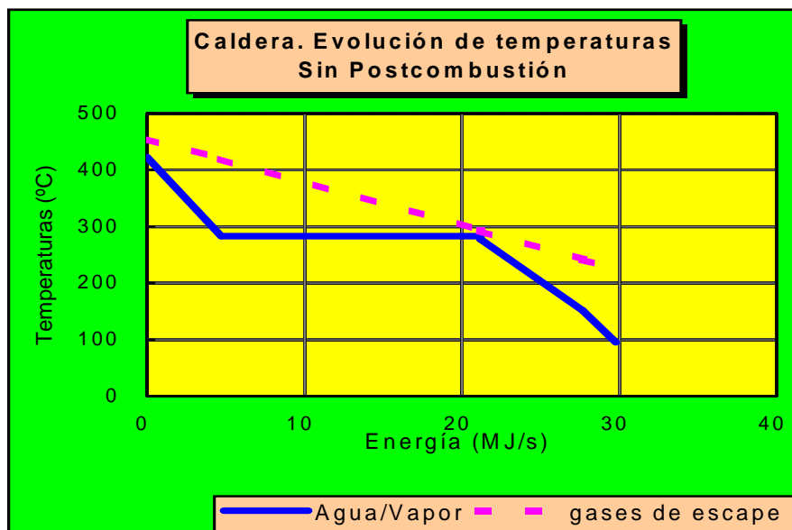
FIG. VIII.3. EVOLUCIÓN DE TEMPERATURAS DE AGUA-VAPOR Y GASES DE ESCAPE, EN UNA CALDERA DE RECUPERACIÓN DE CALOR CON UN NIVEL DE PRESIÓN
