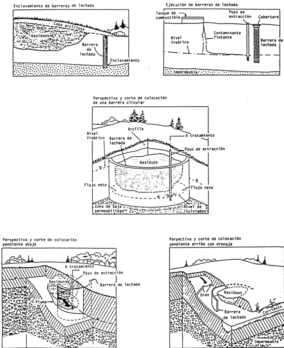
Figura 1. Ejemplos de distintas colocaciones de barreras de lechada
