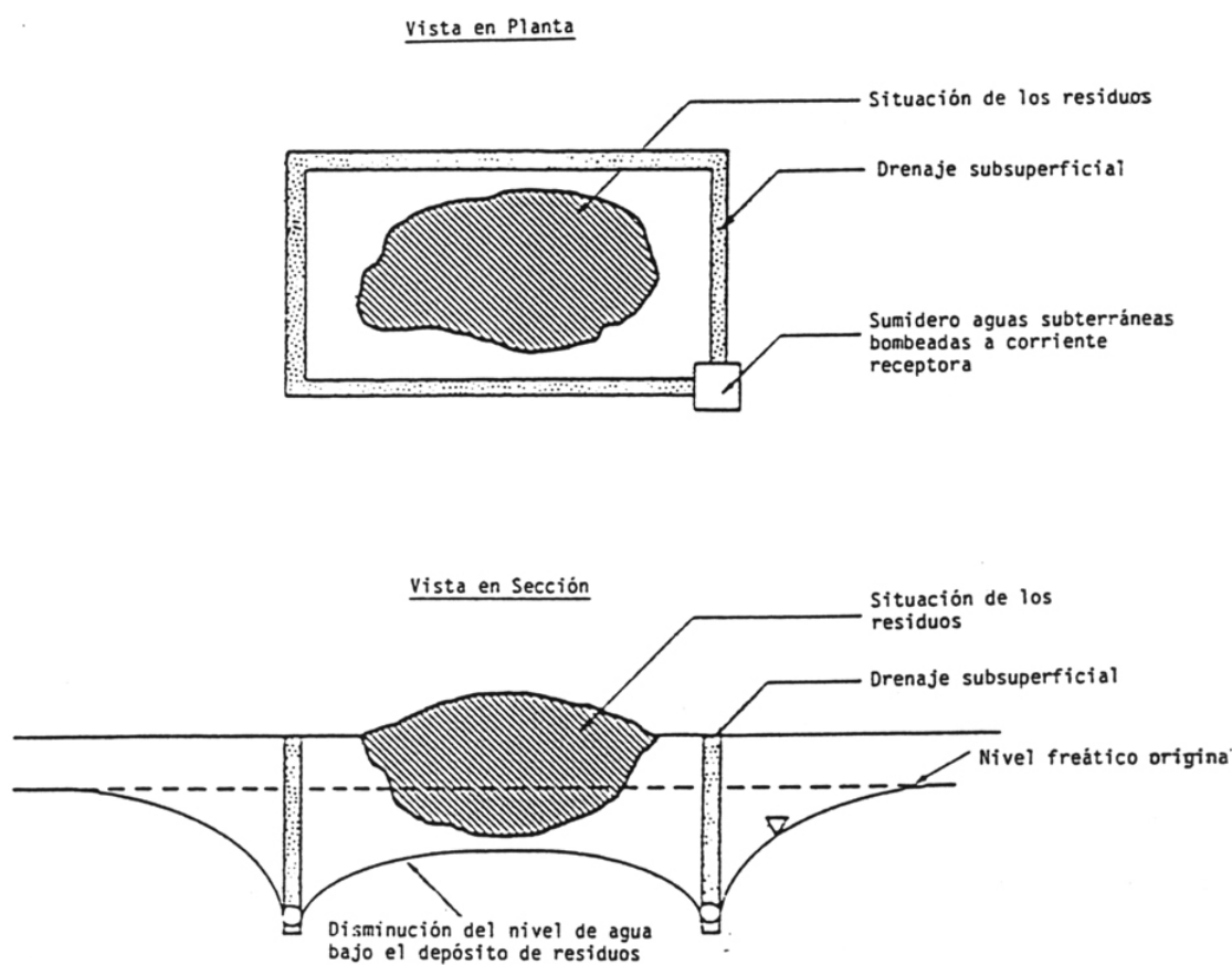
Figura 4. Utilización de drenaje subsuperficial para bajar el nivel freático
