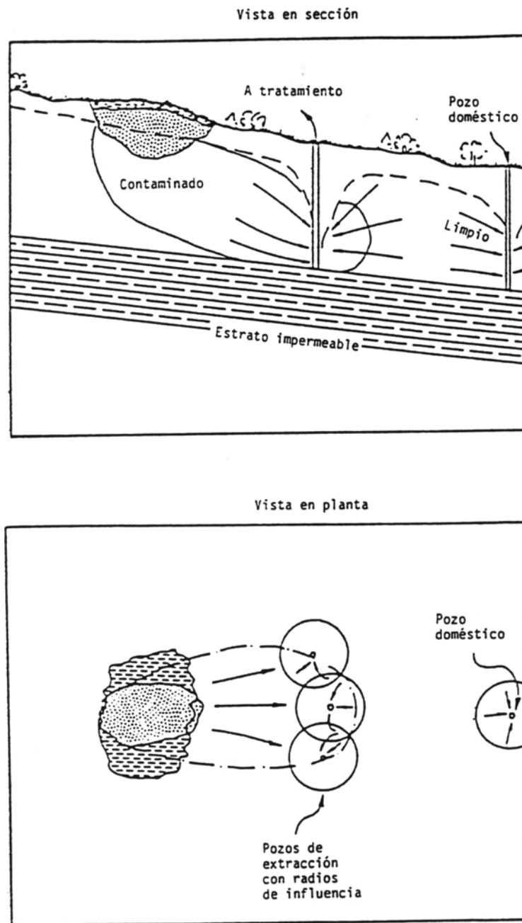
Figura 2. Pozos utilizados para extracción de contaminantes
