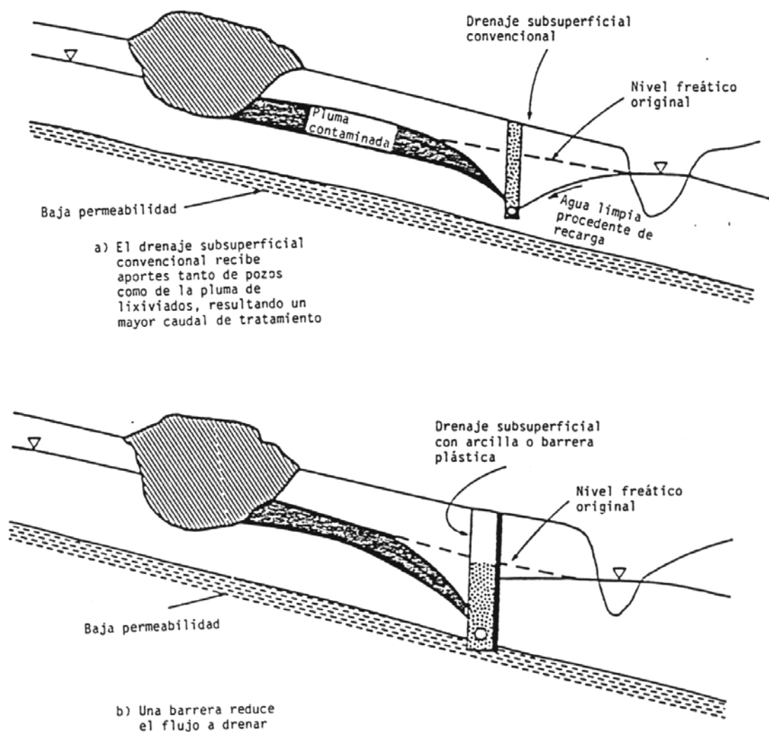
Figura 3. Utilización de drenaje subsuperficial para recoger la pluma de contaminación
